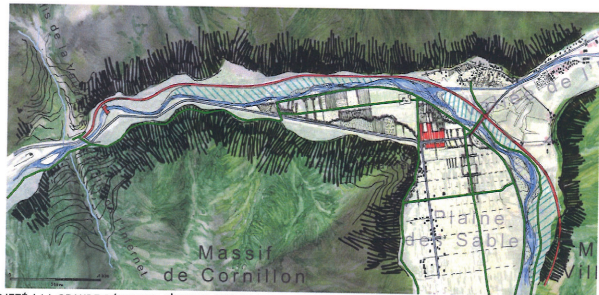
ÉTAT PROJETÉ : LA GRANDE DÉVIATION S'APPUIE SUR LA NOUVELLE DIGUE - LA ROMANCHE EST LIBÉRÉE EN RIVE DROITE
